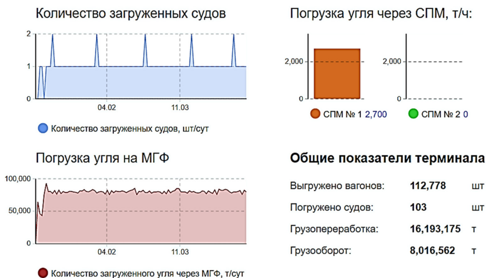
Рис. 9. Интерфейс экрана результатов работы имитационной модели морского грузового фронта терминала (пример)
